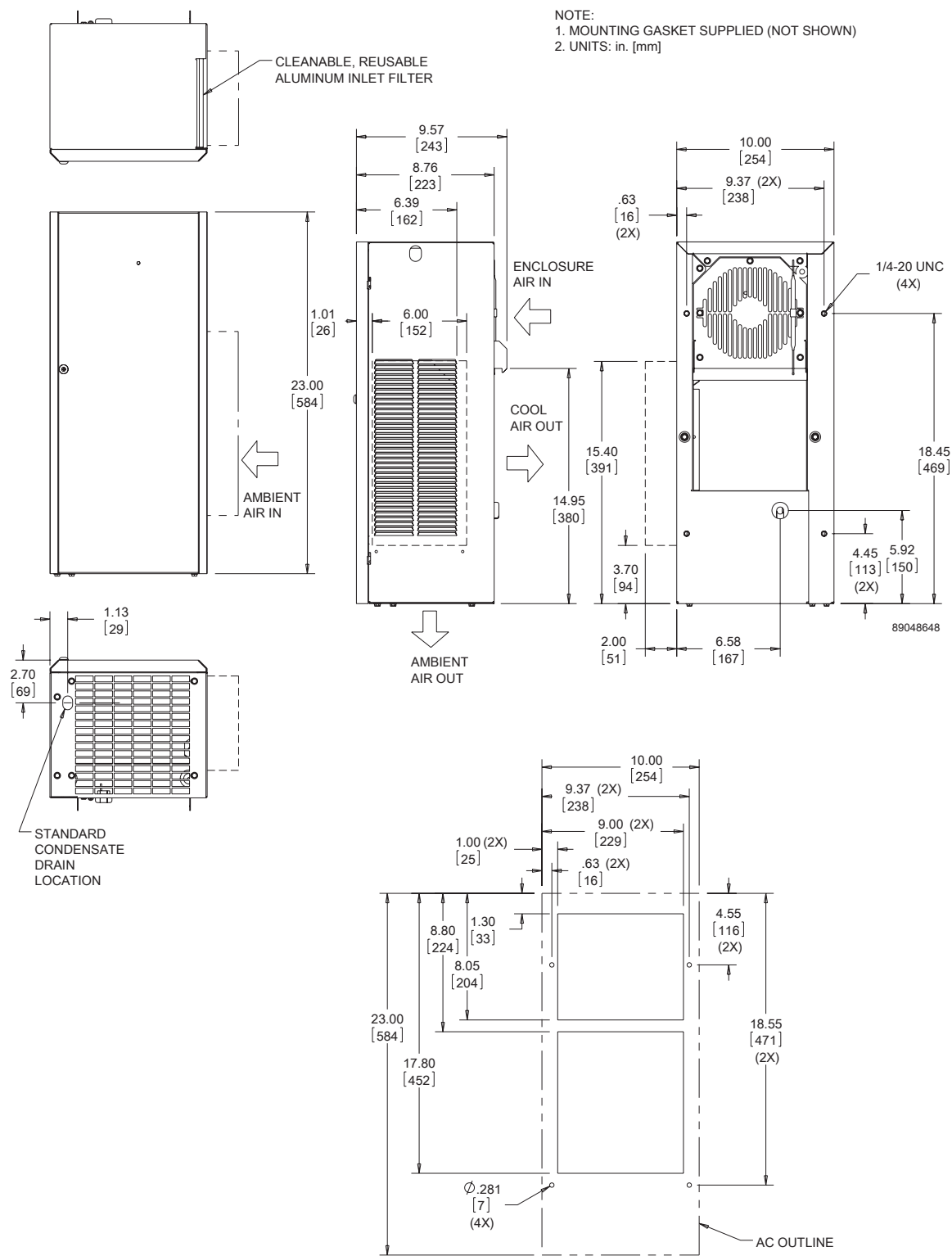
Cutout Dimensions
