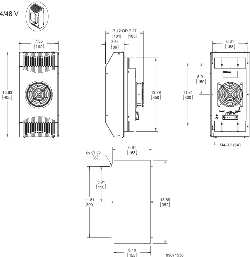
Cutout Dimensions
